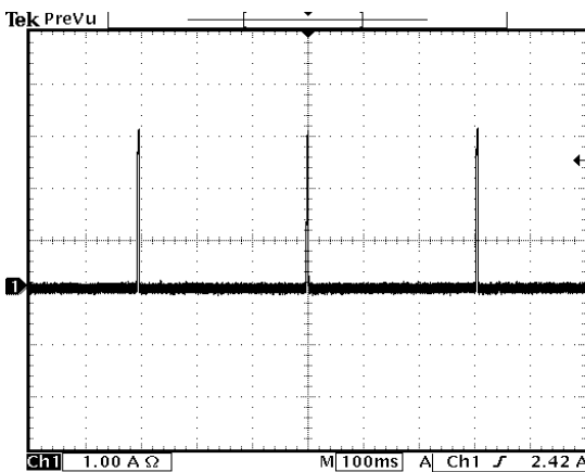
Vin=48V
